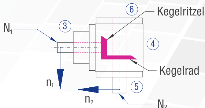
Abbildung 5.3.3-1; Wellenbezeichnungen
