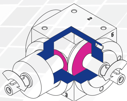
Abbildung 5.3.3-2; Getriebeseiten
