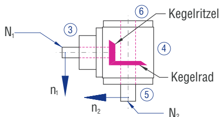
Abbildung 5.2.4-1; Wellenbezeichnungen
